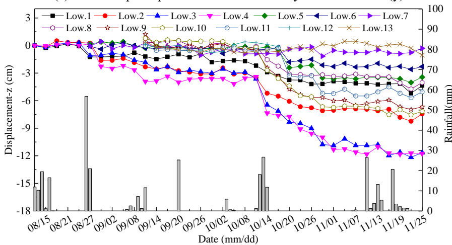
(d) Lower slope settlement deformation (z)
