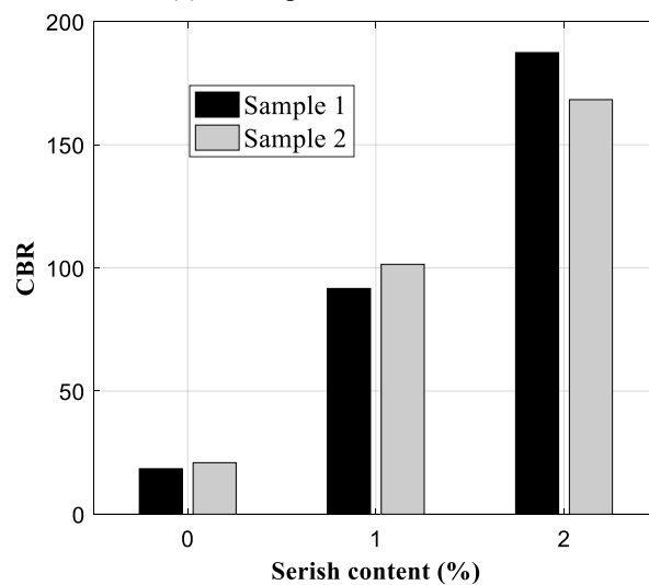
(b) CBR values
