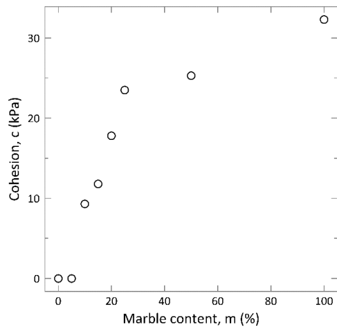
(a) Cohesion
